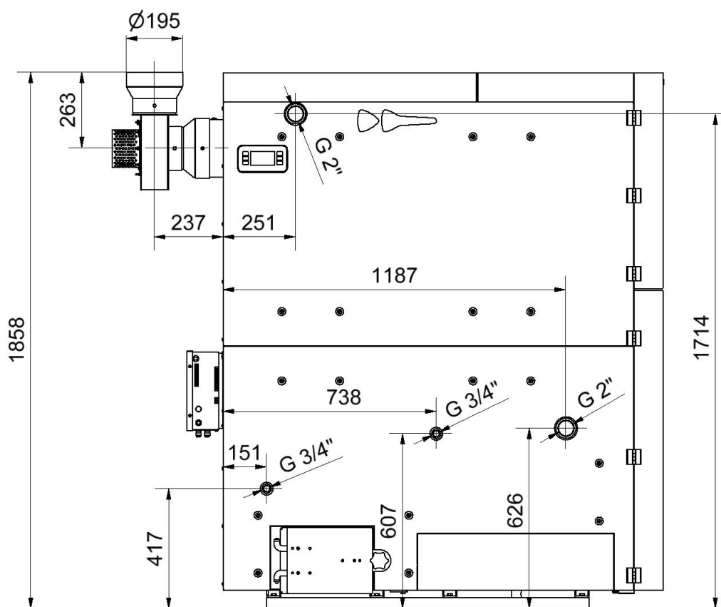
Obr. č. 8 Připojovací rozměry kotle BENEKOV R76
