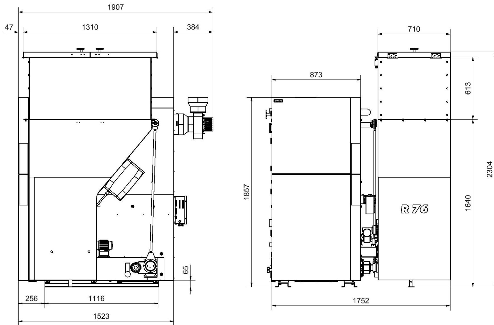
Obr. č. 4 Základní rozměry kotle BENEKOV R76 (s přídatným modulem zásobníku paliva)
