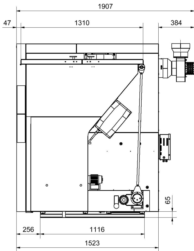
Obr. č. 2 Základní rozměry kotle BENEKOV R76
