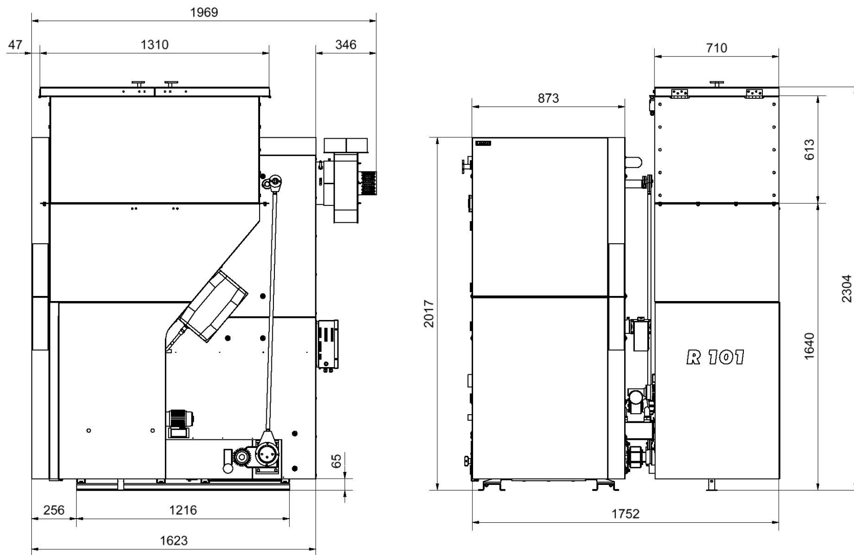
Obr. č. 5 Základní rozměry kotle BENEKOV R101 (s přidavným modulem zásobníku paliva)
